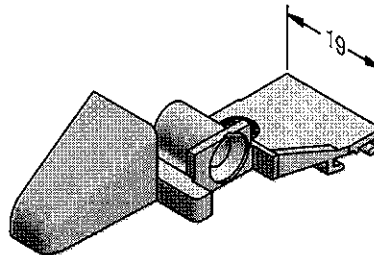
Endkappe Wetterschenkel 15 ED86 plus ASA
