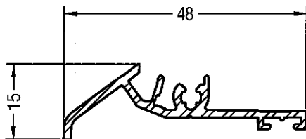
Wetterschenkel 15 ED86 plus
