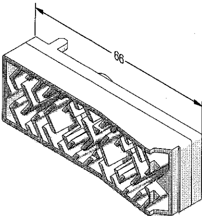
Windstopp ED86 plus ASA/TPE
